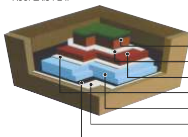
ACOPERIS PLAT
